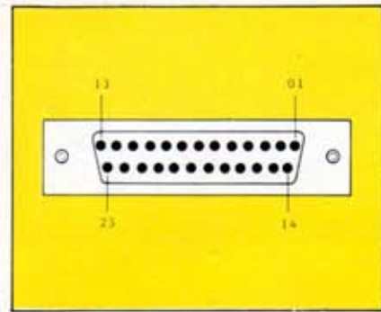
Figura 2 — Conector (Padrão ISO 2110-1980)
